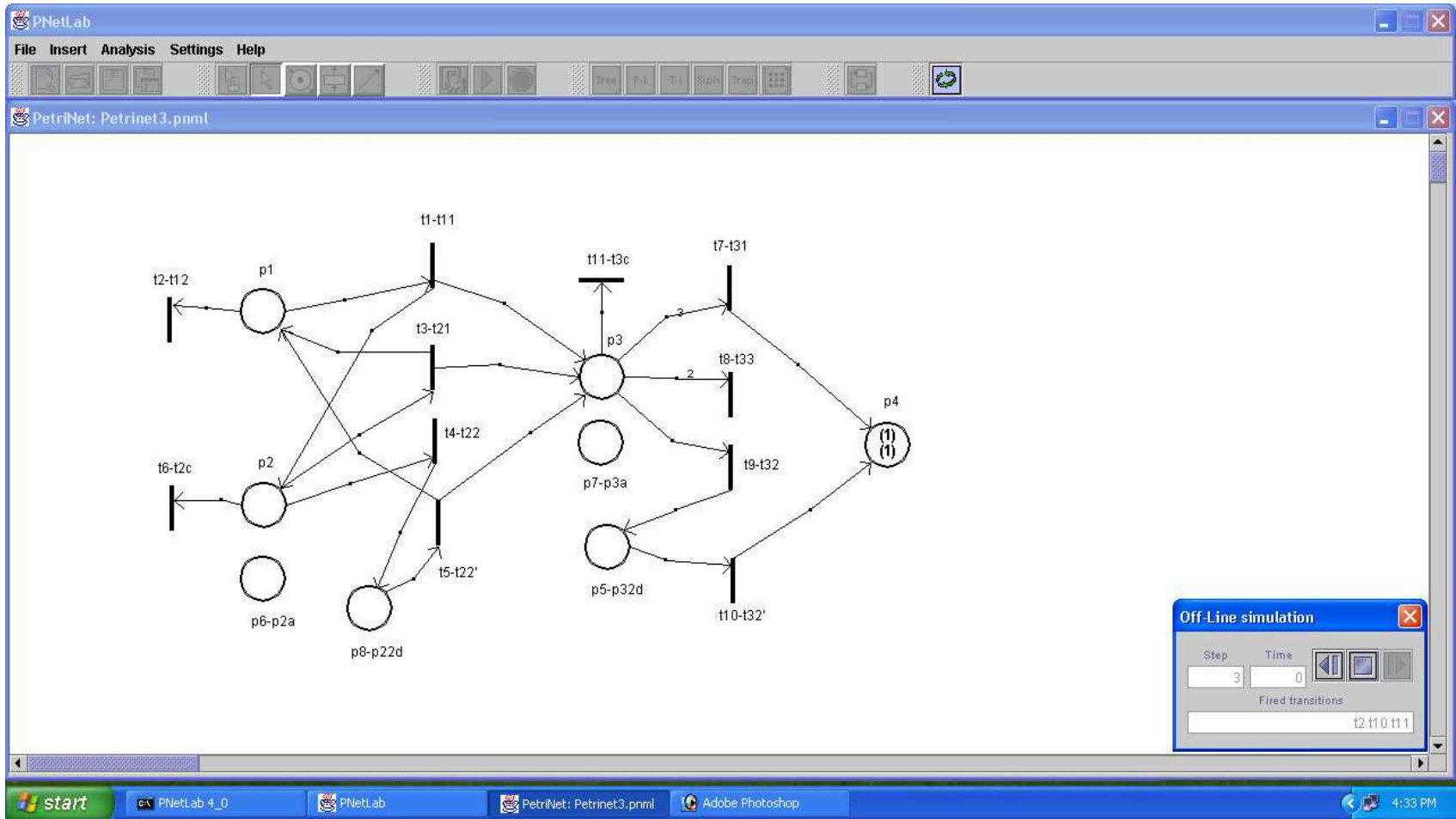
(d) Simulation of \mathcal{NL}_{\Pi_1} in PNetLab (Step 4)
